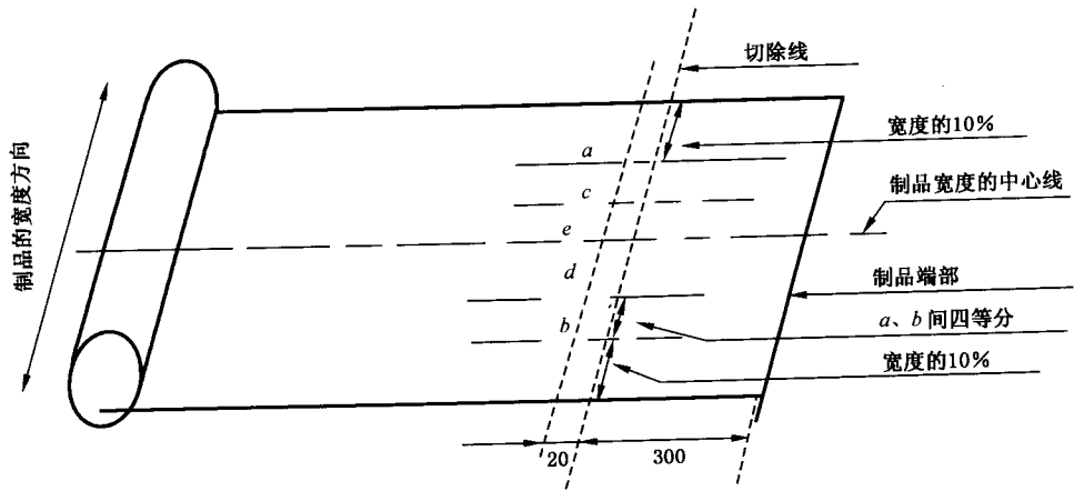
图 1 厚度测量点示意图
