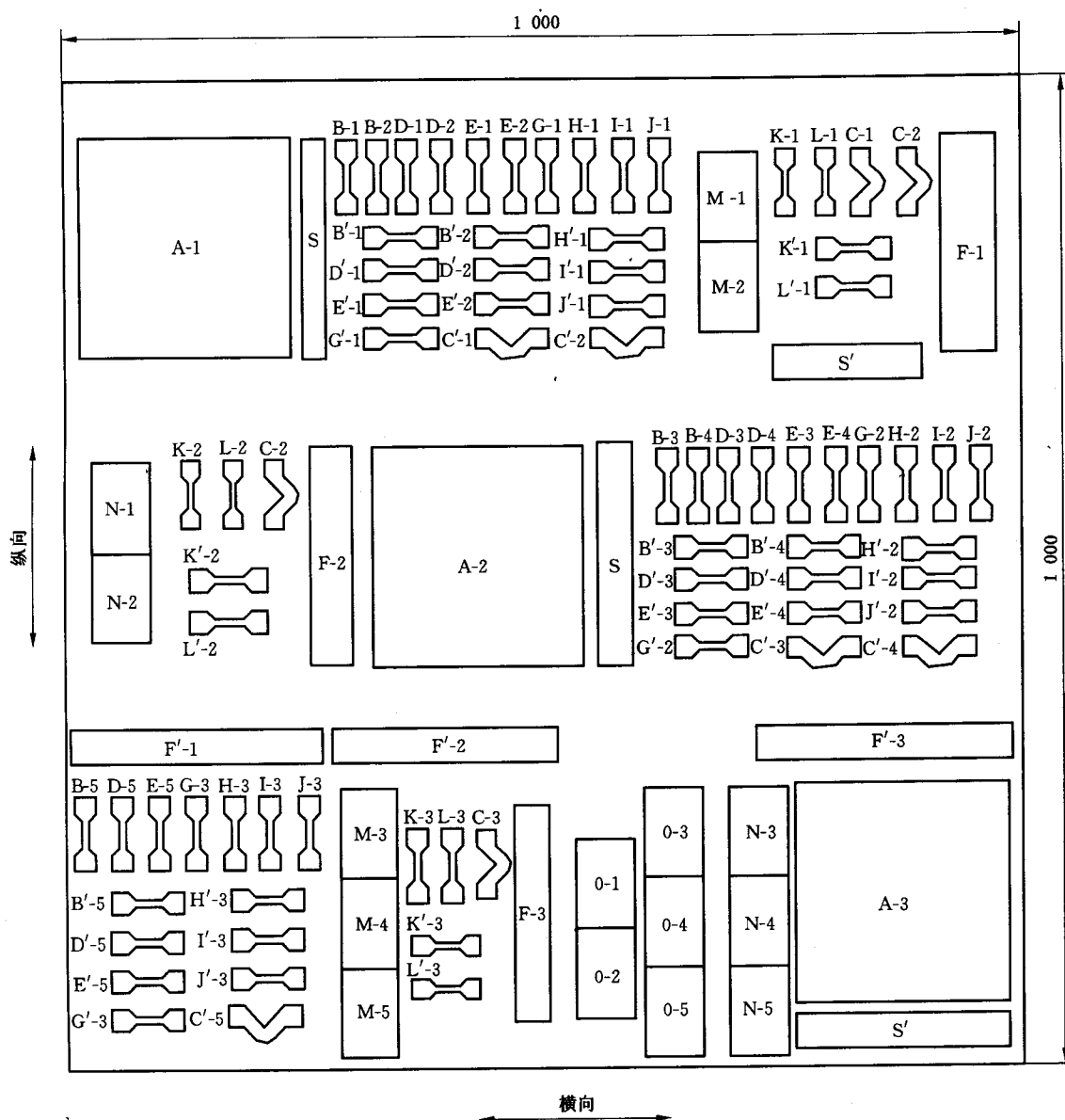
图 2 裁样示意图
