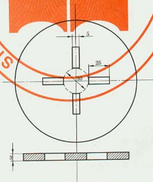
图 3 透水仪压板示意图
